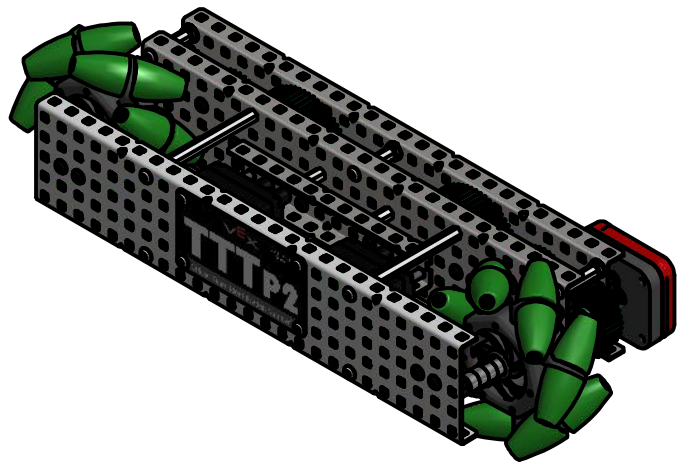
V. Chasis Derecho ESCALA 1 / 4
