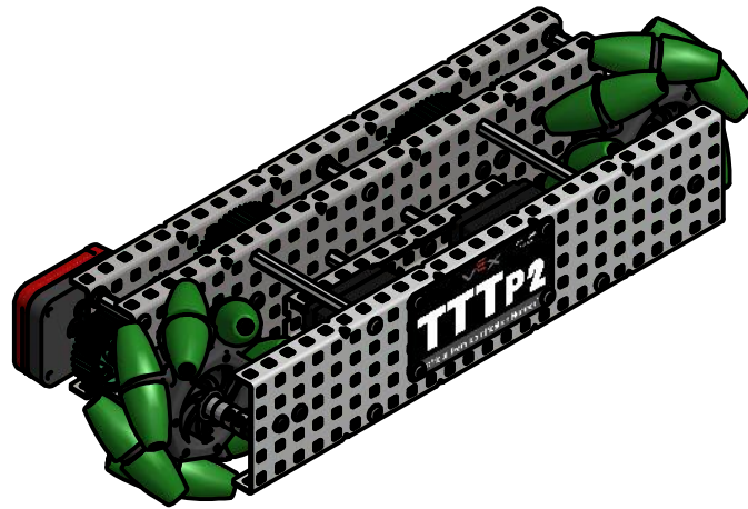
V. Chasis Izquierdo ESCALA 1 / 4
